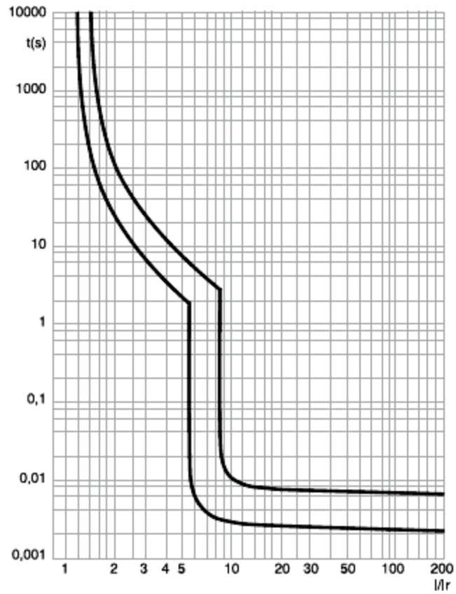
Curva característica de intervención C
