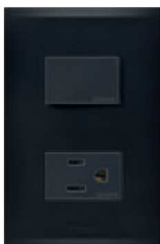
FZ2231N Placa con 1 interruptor sencillo 15A 127V y 1 tomacorriente 2P+T 15A 127V.
